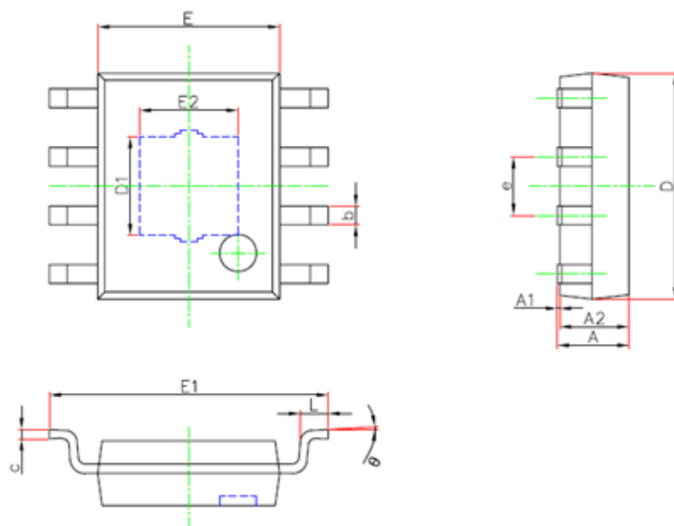
8引脚ESOP封装（单位mm）
