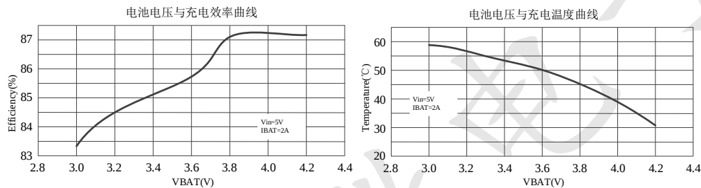
电池电压与充电效率曲线
