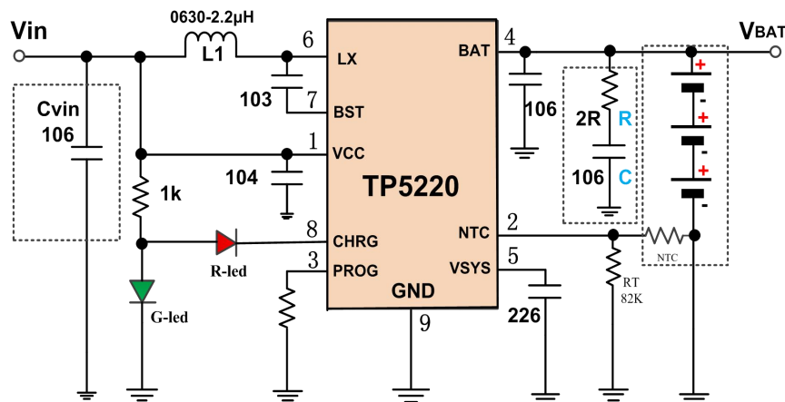
应用四：TP5220 双灯 3 节充电应用示意图
