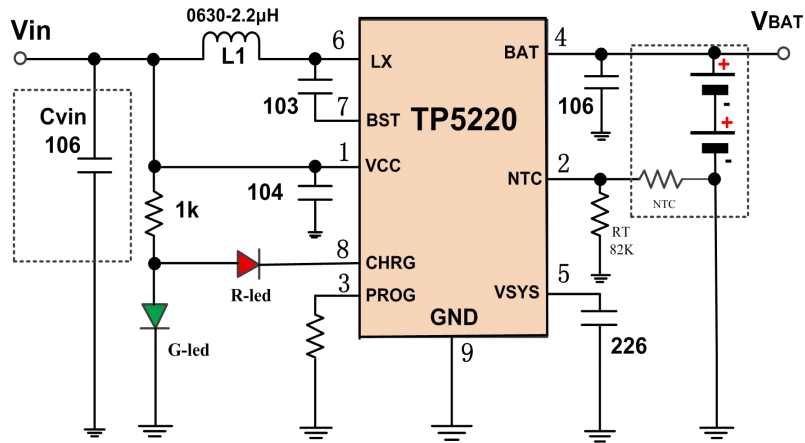
应用二：TP5220 双灯 2 节充电应用示意图
