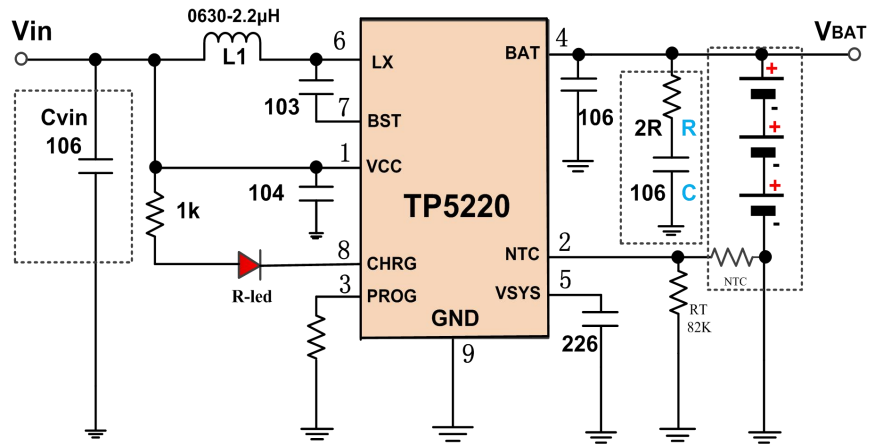
应用三：TP5220 单灯3节充电应用示意图
