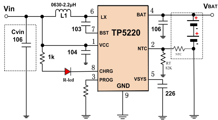
应用一：TP5220 单灯2节充电应用示意图
