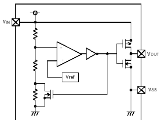
(1) CMOS Output
